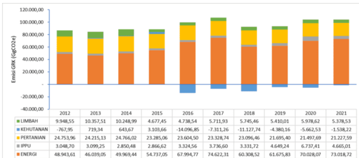
Gambar 2.20 Perkembangan Emisi GRK di Provinsi Jawa Tengah (GgCO 2 e)
