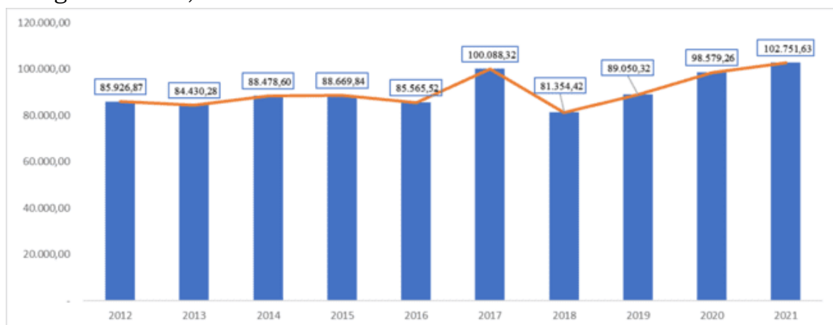
Gambar 2.19 Tingkat Emisi GRK Provinsi Jawa Tengah Tahun 2012-2021
